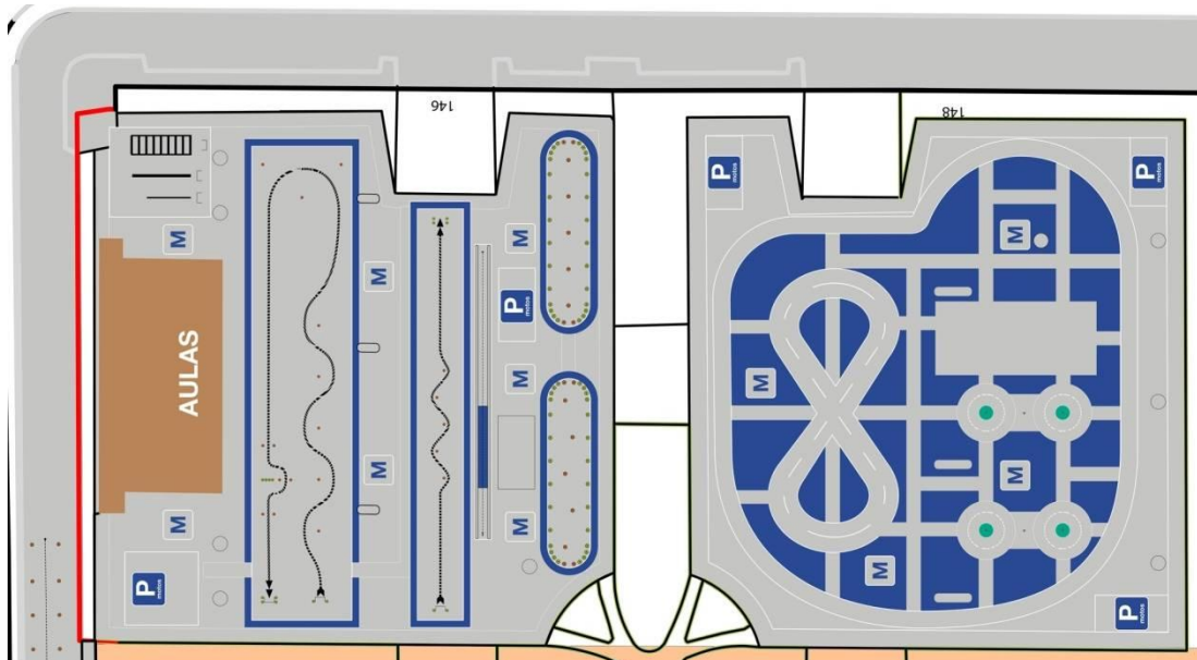
Plataforma dinámica asfaltada de 12.000 m 2 .
